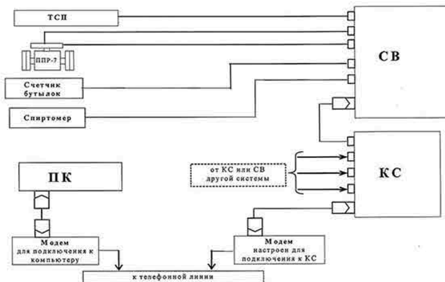
Рисунок 2 - Схема соединений составных частей системы
